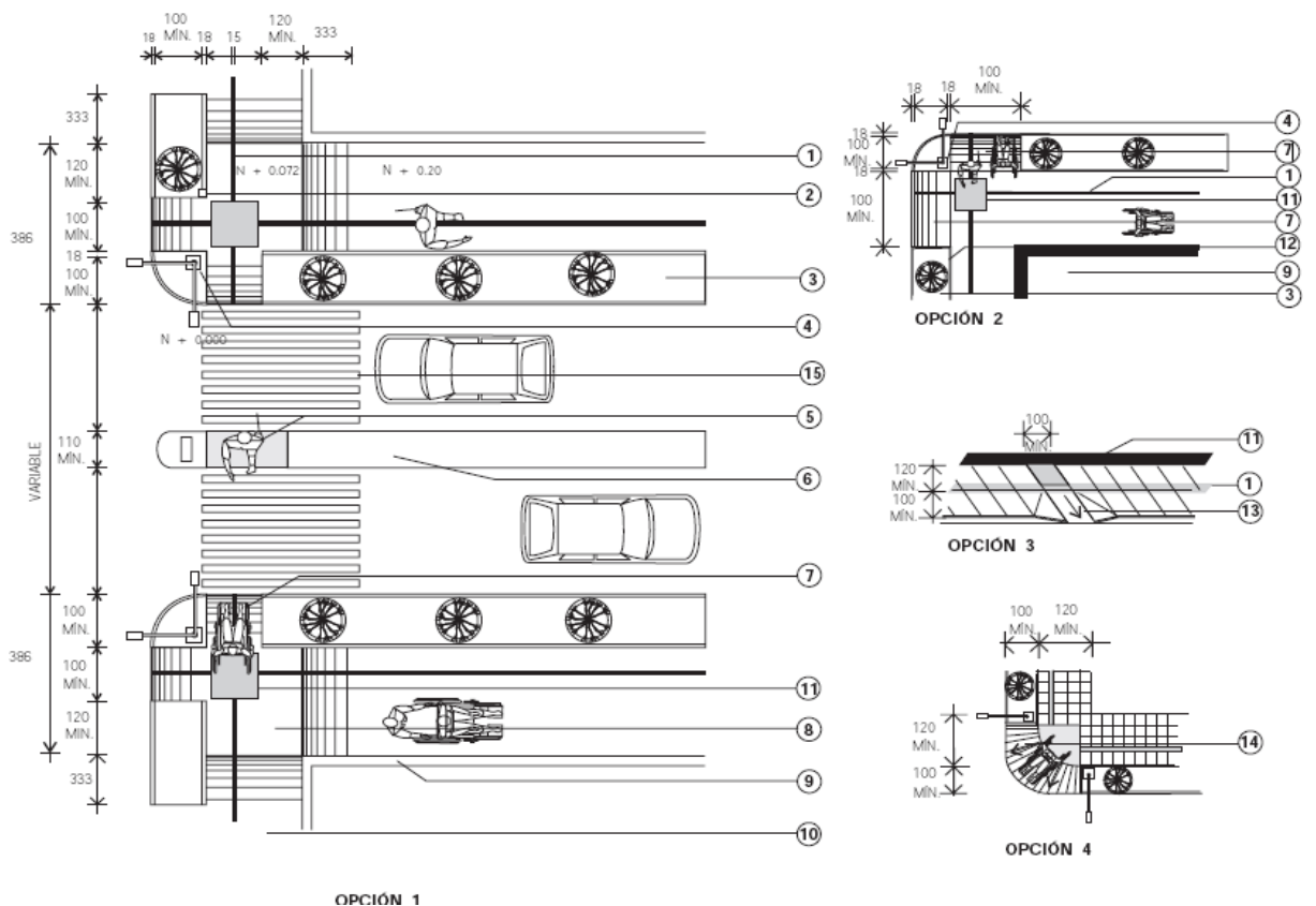
Planta
