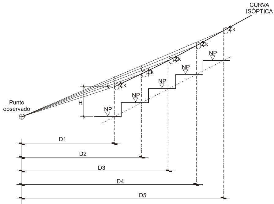
Figura 5.1.- Trazo de la Isóptica (Ilustrativa)
