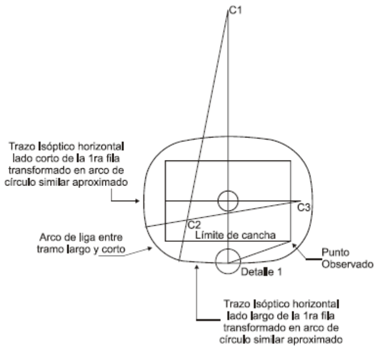
Figura 5.3.- Trazo de la Isóptica Horizontal (Ilustrativa)
