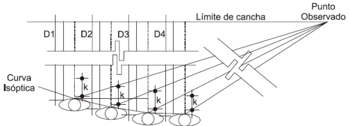
Figura 5.4.- Trazo de la Isóptica Horizontal (Ilustrativa)
